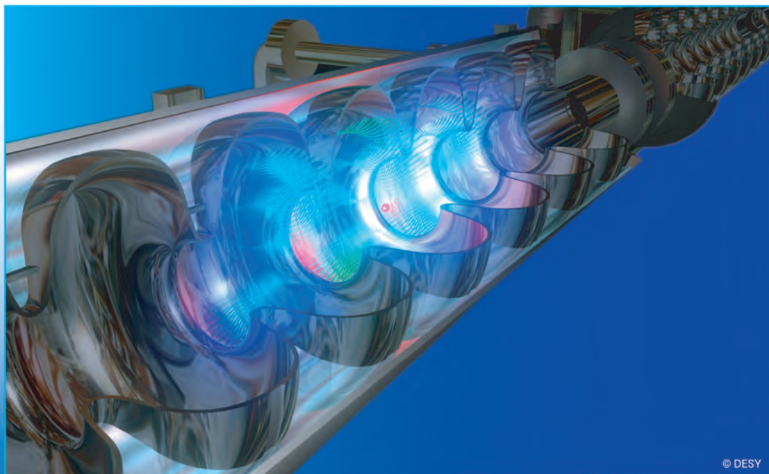
European XFEL: Electromagnetic fields accelerating electrons in superconducting resonators European XFEL: Электромагнитные поля, ускоряющие электроны в сверхпроводящих резонаторах
